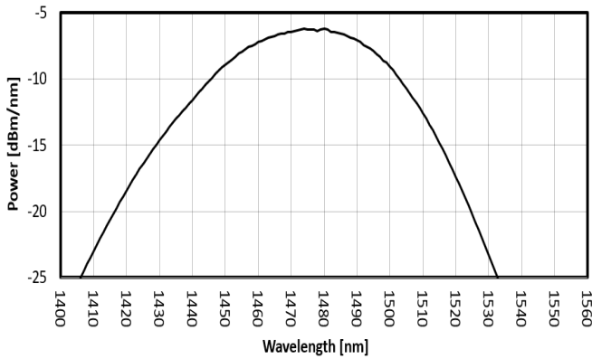
FIG. 1: ISB1 SPECTRUM
