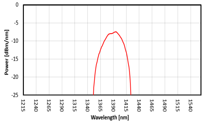
FIG. 4: SLED 3 SPECTRUM
