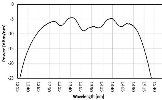
FIG. 1: ISB2 SPECTRUM
