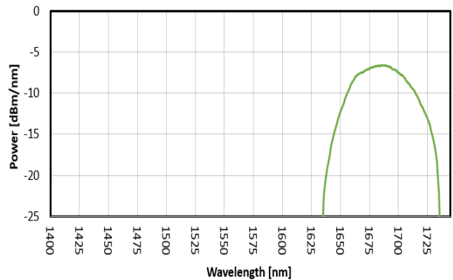
FIG. 2: SLED 1 SPECTRUM
