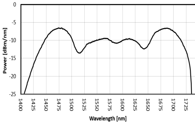
FIG. 1: OSE2 SPECTRUM
